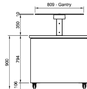
End Elevation
